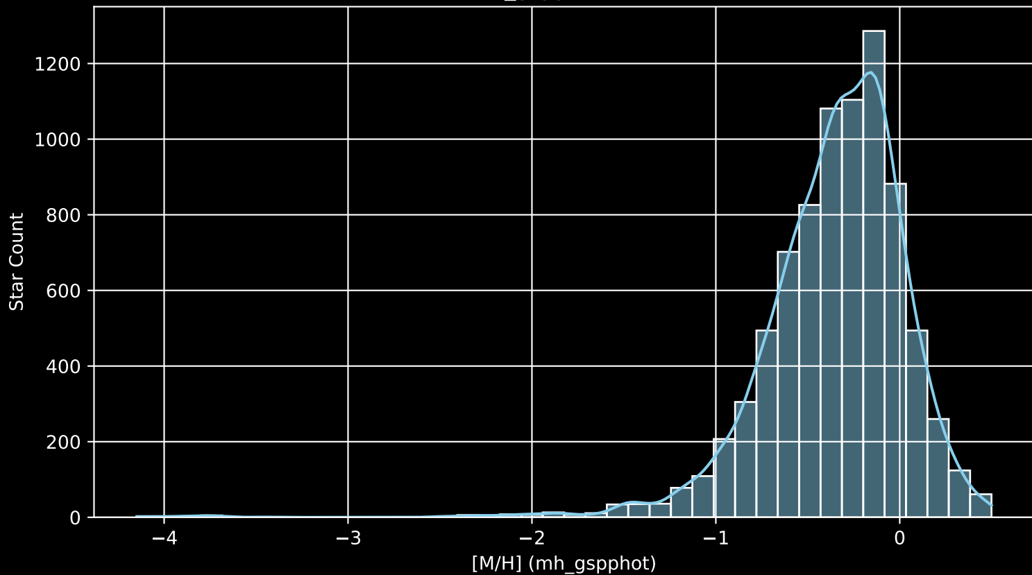
GALAH DR4 Field: [-5] [M/H] (mh_gspphot) (n= 8192)
