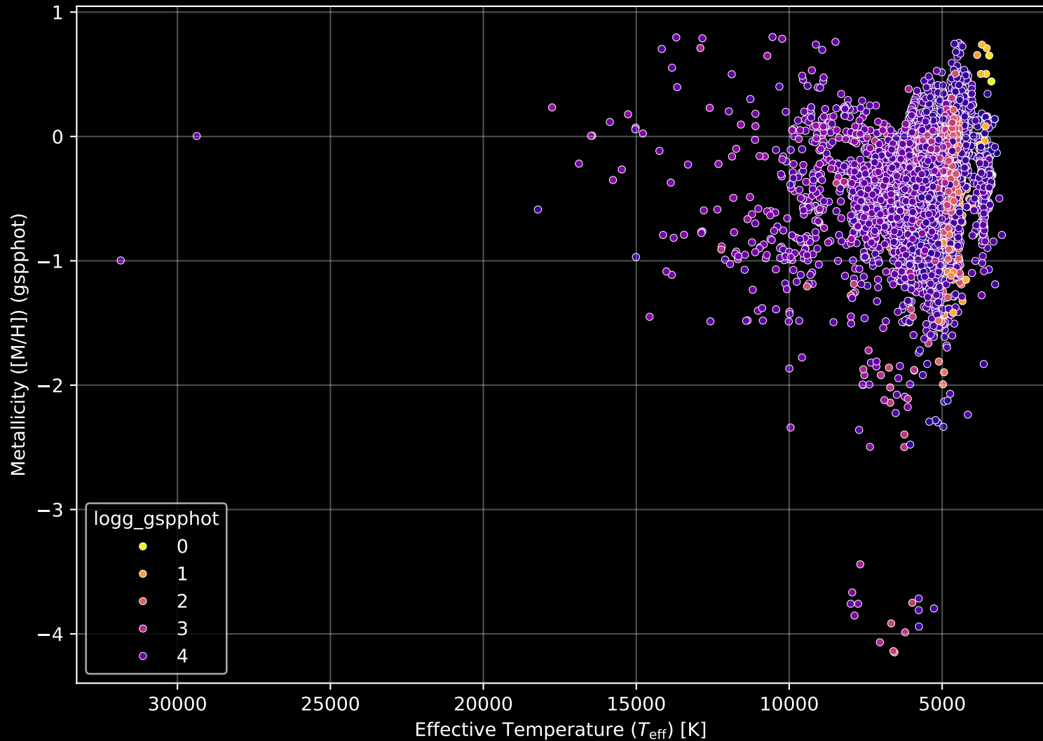
GALAH DR4 Field: [-5] Stellar Population Parameters (n= 8235)
