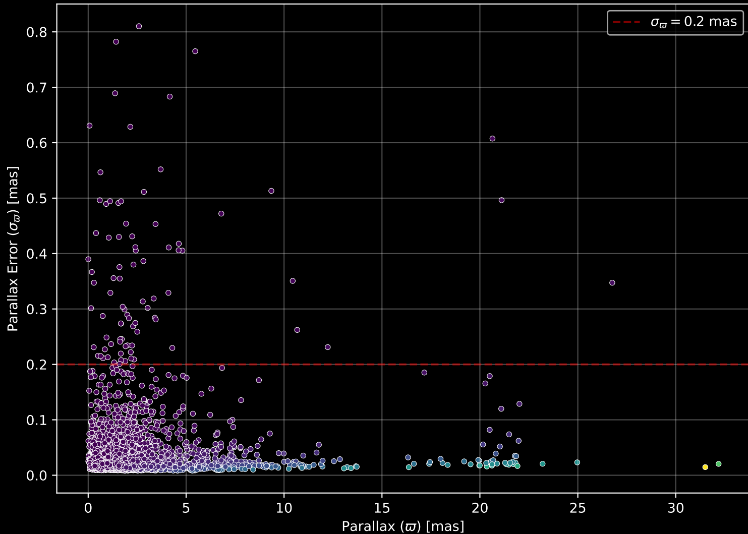
GALAH DR4 Field: [-5] Parallax Quality (n= 8235)
