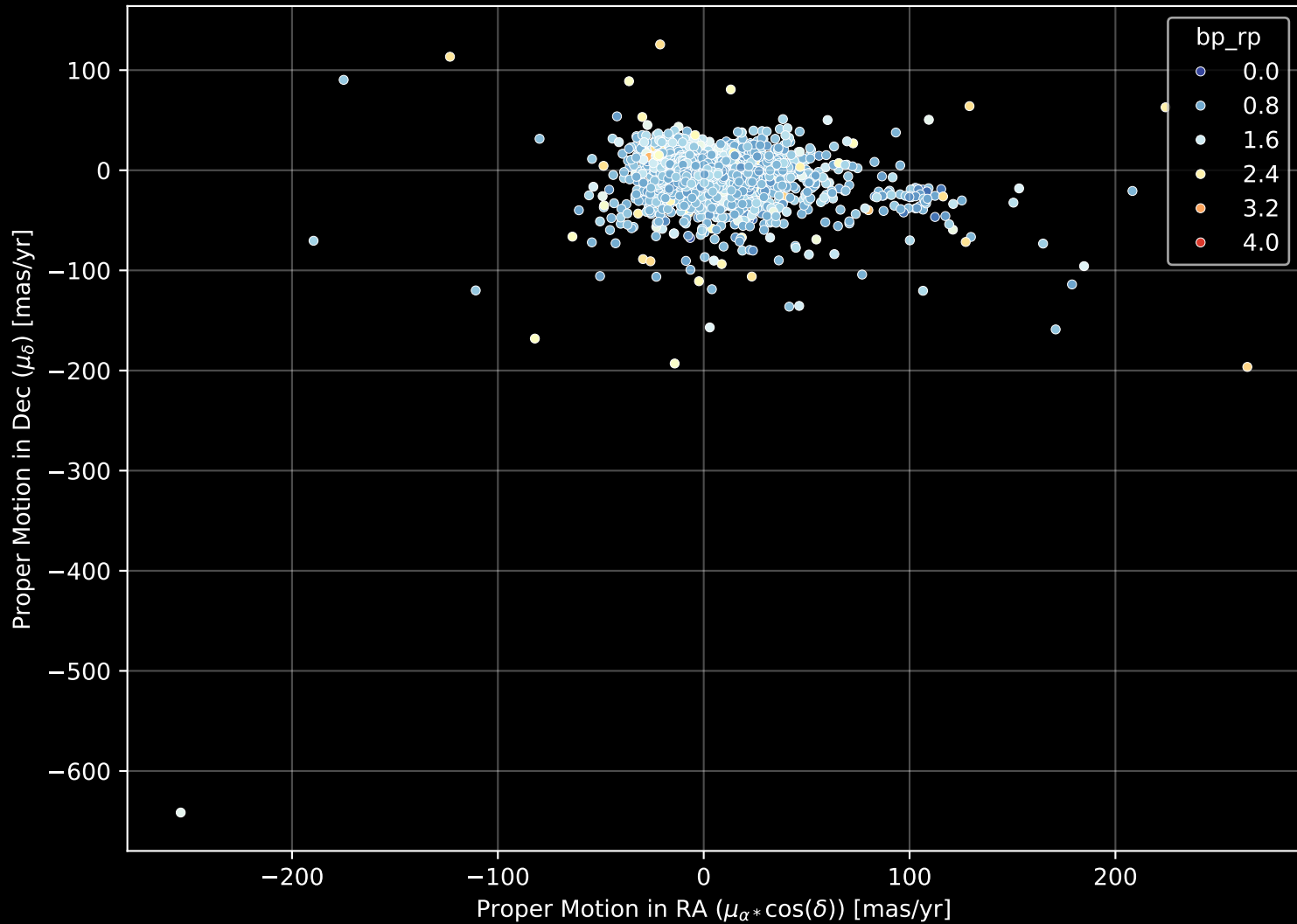
GALAH DR4 Field: [-5] Proper Motion Diagram (n= 8235)
